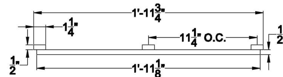
ELEVATION B
