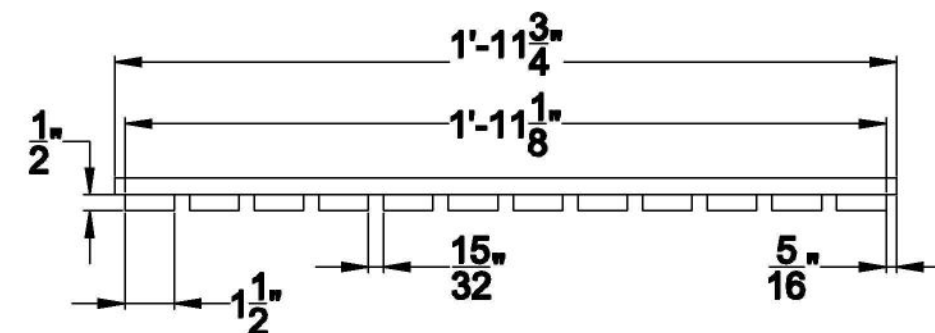
ELEVATION A
